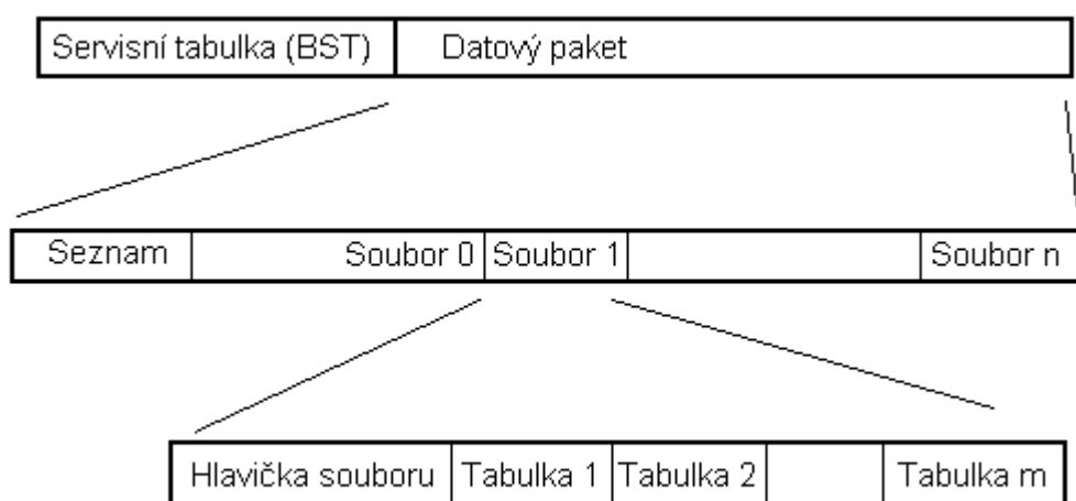
Obrázek 1 – Schéma skladby datové komunikace
