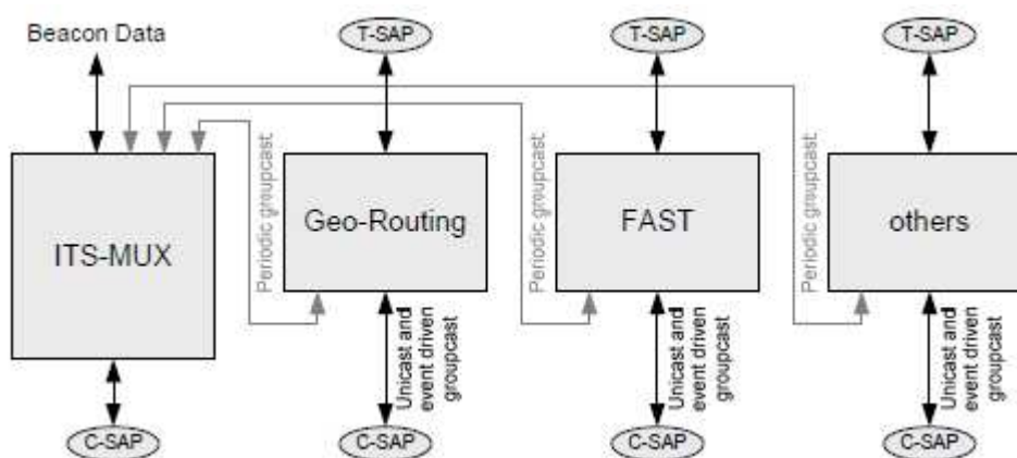
Obrázek 13 – Architektura protokolu ITS-MUX
