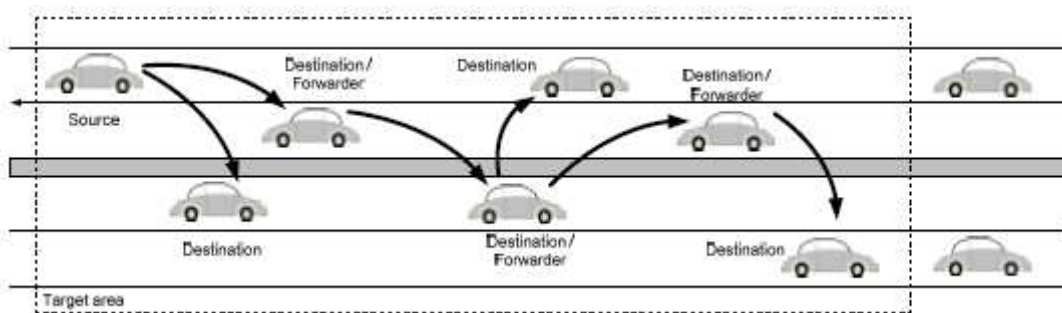
Obrázek 5 – Metoda Geo-broadcast
