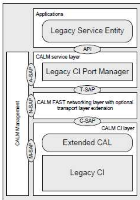
Obrázek 1 – Struktura komunikačního modulu FAST CALM
