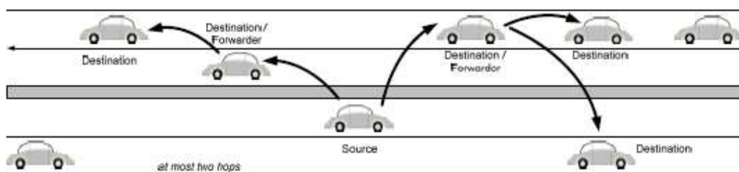
Obrázek 7 – Metoda N-hop broadcast
