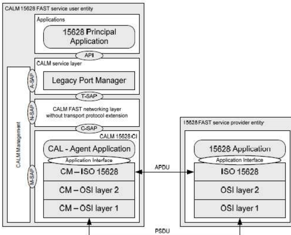
Obrázek 17 – Architektura systému CALM s Agentem aplikací
