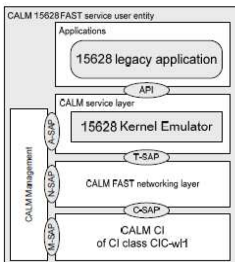
Obrázek 2 – Uživatelská aplikace na 15628 DSRC platformě
