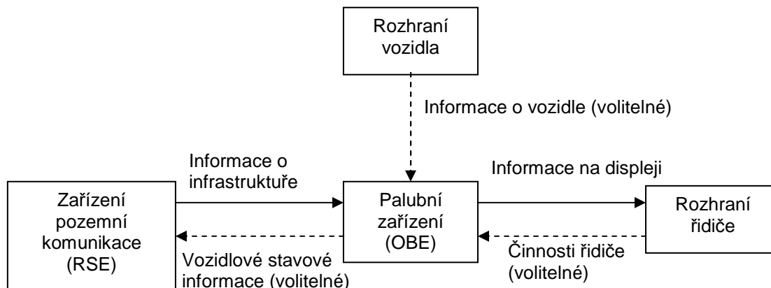
Obrázek 1: Uspořádání systému
