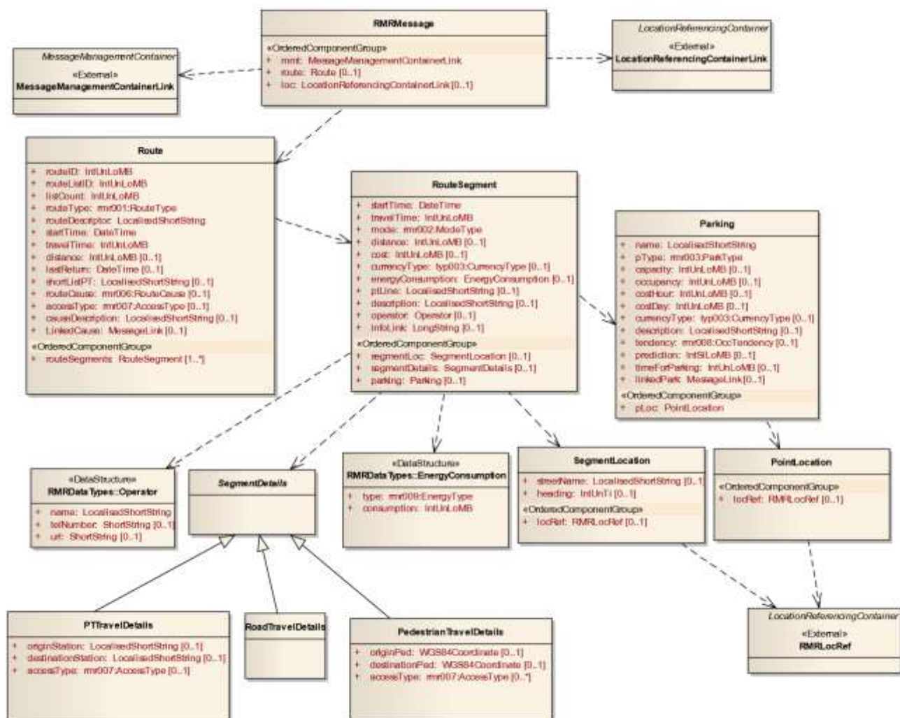
Obrázek 1 - UML model tříd aplikace RMR (obrázek 2 normy)
