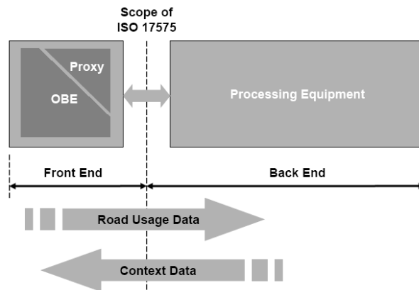
Obrázek 2 – Předpokládaná technická architektura a rozhraní
