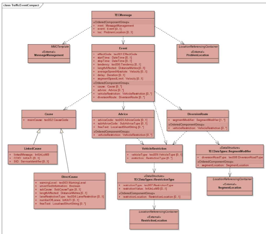
Obrázek 1 UML model TPEG-TEC
