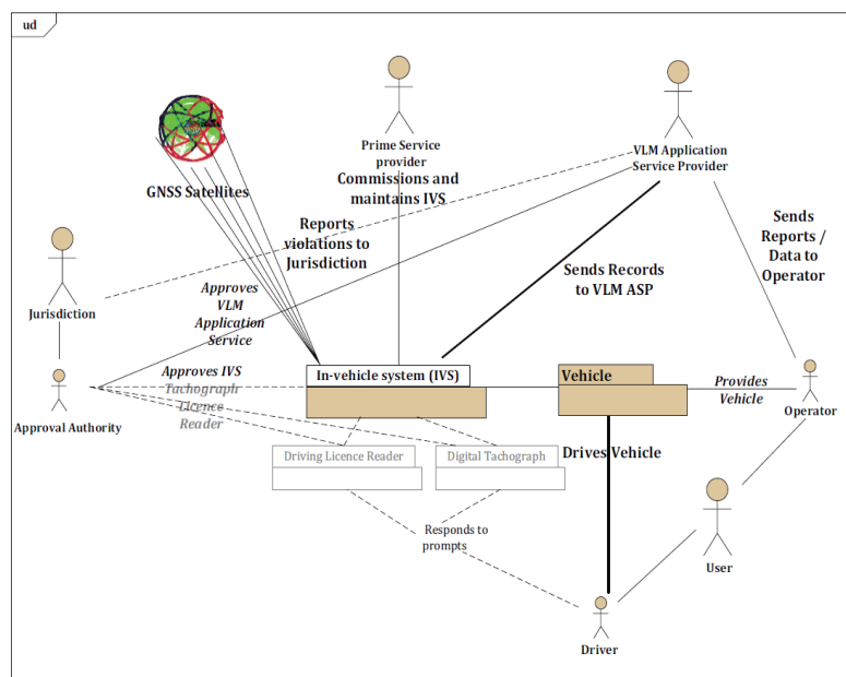
Obrázek 1 – Příklad užití TARV VLM (obr. 2 normy)
