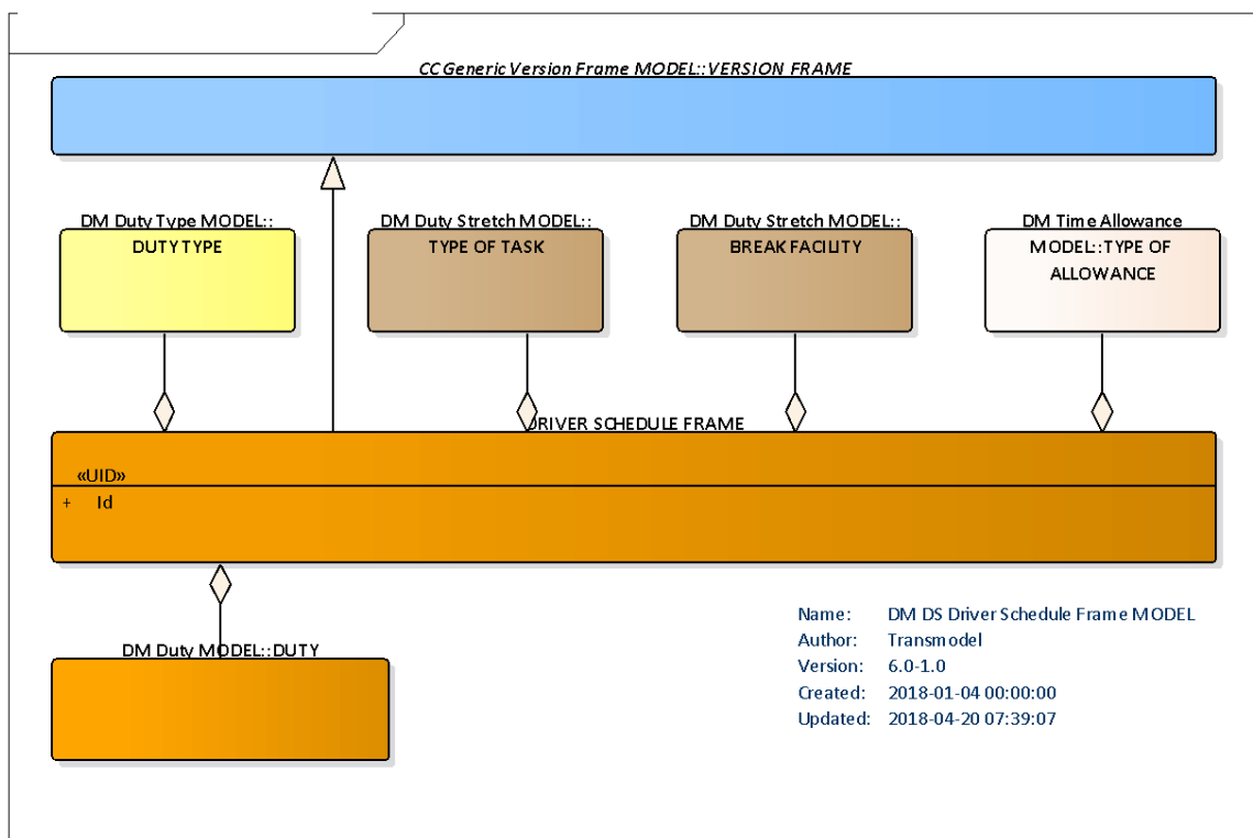
Obrázek 1 – UML model tříd – Rozpis řidiče (obr. 8 normy)
