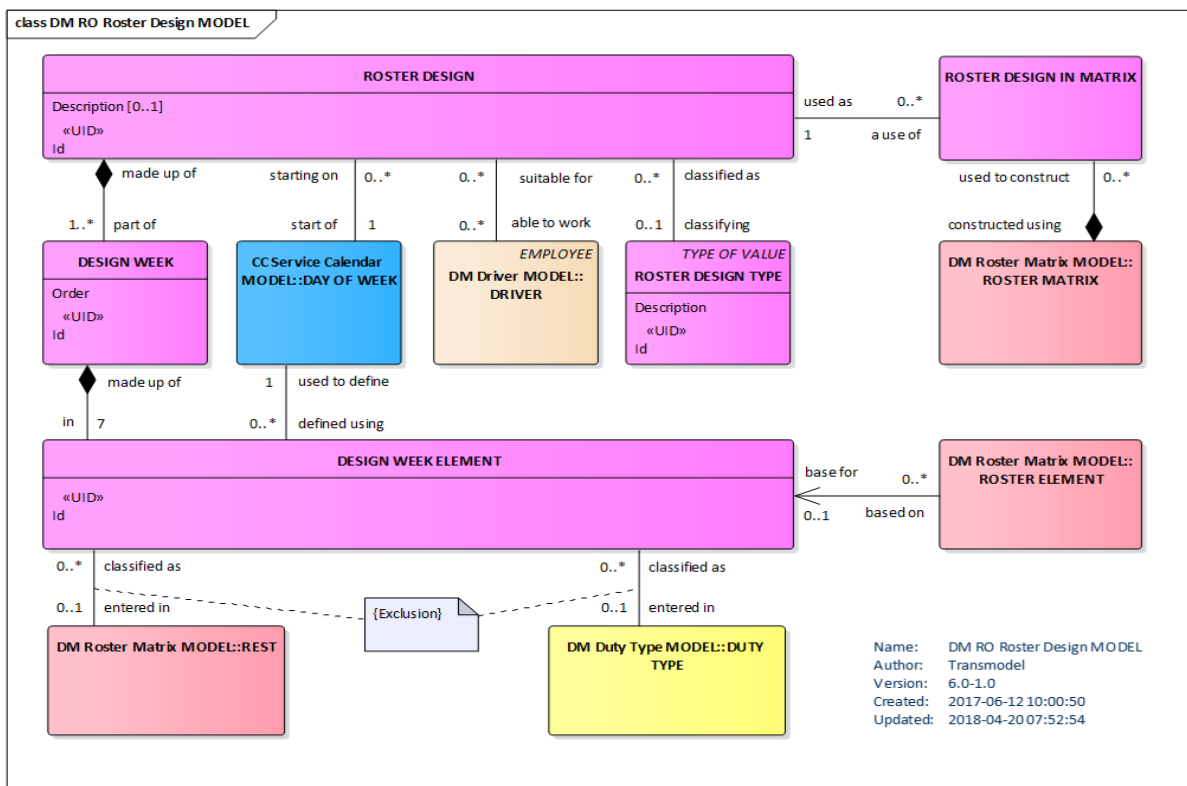
Obrázek 2 – UML model - Matice přiřazení povinností (obr.18 normy)
