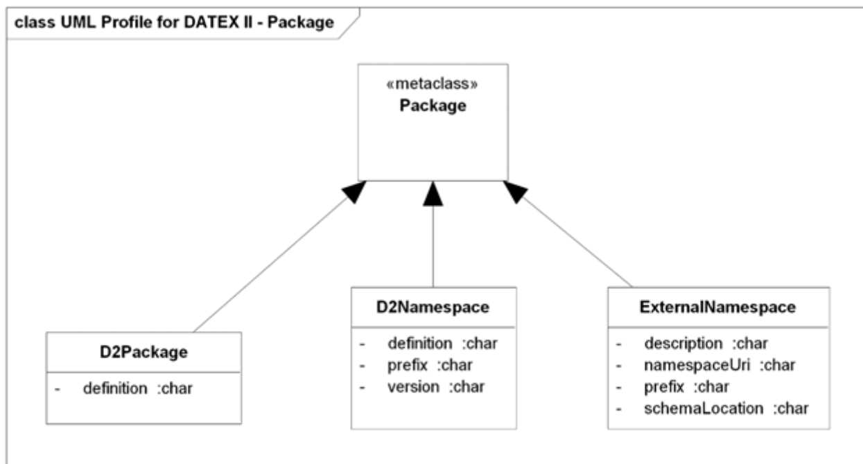
Obrázek 3: Balíčky (obr. 8 popisovaného dokumentu)
