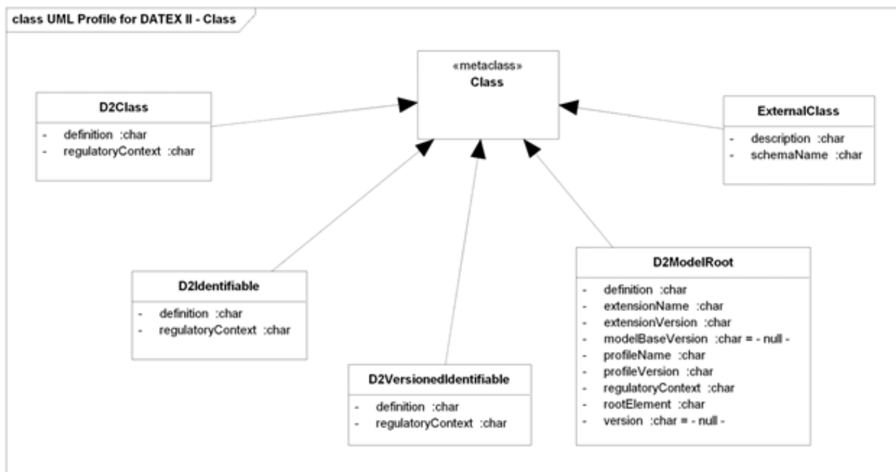
Obrázek 2: Třídy (obr. 3 popisovaného dokumentu)
