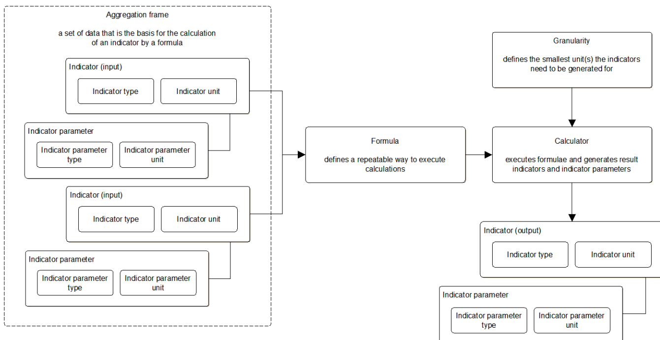
Obrázek 1 –Výpočet indikátorů referenční model (obr.1 normy)
