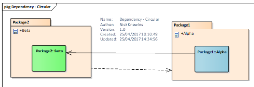
Obrázek 3 – Závislosti balíčků a tříd (obr. B.12 normy)
