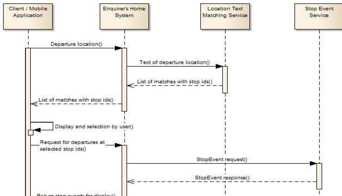
Obrázek 2 – Sekvenční diagram pro monitorování odjezdu (obr. 2 normy)
