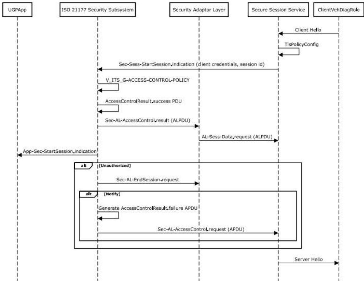
Obrázek 6 (obrázek 16 normy): Sekvenční diagram zahájení TLS session
