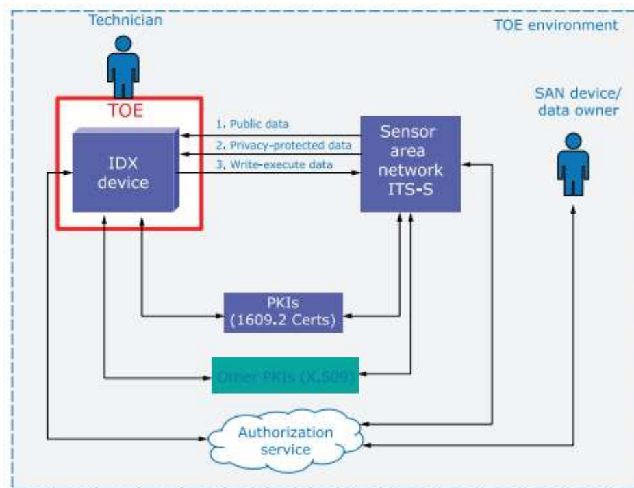
Obrázek 1 (obrázek 8 normy): Systémový pohled na "cíl vyhodnocení"
