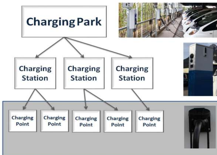
Obrázek 1 - Struktura nabíjecí infrastruktury (Obrázek 2 normy)
