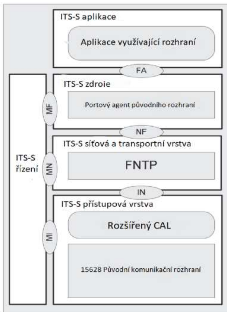
Obrázek 1 (obr. 3 normy) – Architektura stanice ITS s původním rozhraním podle ISO 15628
